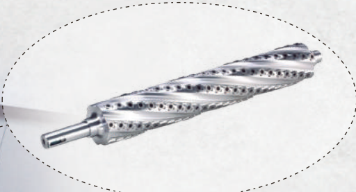
EJE HELICOIDAL HELICAL SHAFT ARBRE HÉLICOÏDAL
