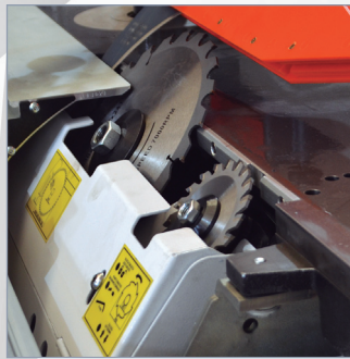
Grupo sierra e incisor Saw blade and scoring group Groupe disque et inciseur
