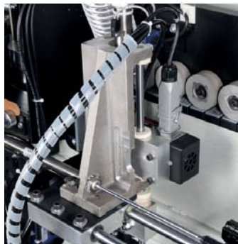
Grupo retesteador (doble disco) End cutting unit (two blades)
