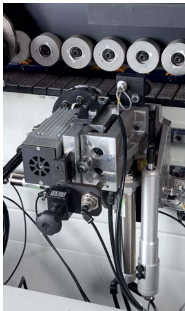
Grupo ribeteador Rounding unit
