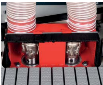
Grupo rectificador (doble tupi) Pre milling unit (two tools)
