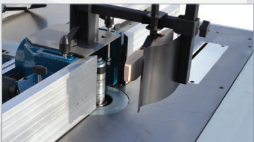
Tupi Spindle moulder Toupie
