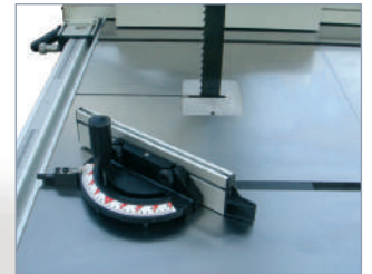
Guía de ángulos Miter fence Guide d'angles
