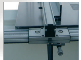
Palograma milimétrico Milimetric fence Guide milimétrique
